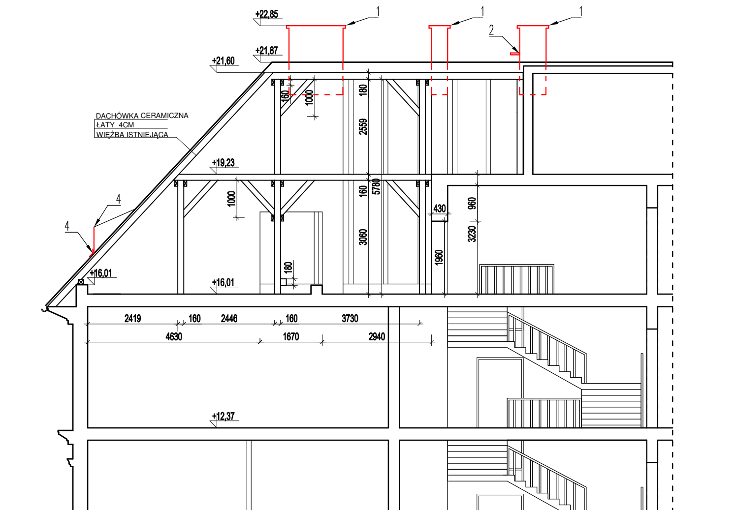
PRZEKRÓJ C-C
